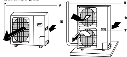
Универсальный внешний блок EACO-48H/UP2/N3, EACO-48H/UP2/N3_LAK, EACO-60H/UP2/N3, EACO-60H/UP2/N3_LAK
