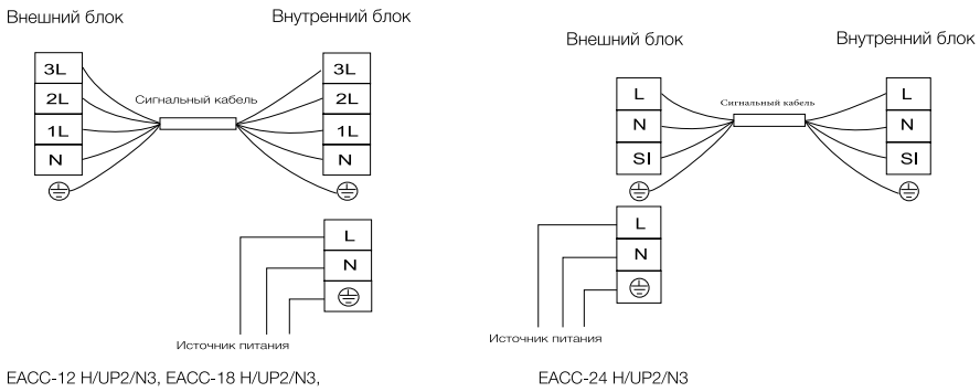
EACC-12 H/UP2/N3, EACC-18 H/UP2/N3,
